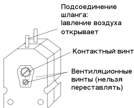
Выключатель давления
